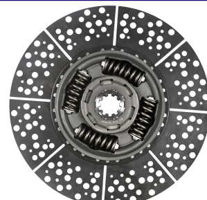
VW 24280 MOTOR MAN 4 MOLAS 10 ESTRIAS 395MM (SACHS 5638)
