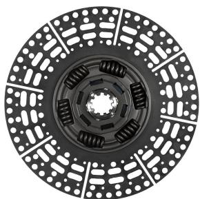
VW TITAN COM PRÉ DAMPER 6 MOLAS 10 ESTRIAS 380MM (SACHS 5383)
