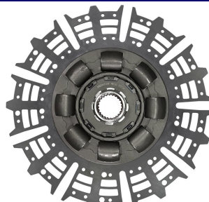
SCANIA 124 C/ PRÉ-DAMPER 8 MOLAS 24 ESTRIAS 430MM (SACHS 5453)
