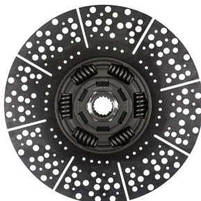
MB 1722 C/ PRÉ-DAMPER 4 MOLAS 18 ESTRIAS 395MM (SACHS 5766)
