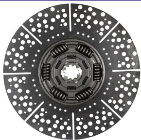
VW CONSTELLATION C/ PRÉ DAMPER 6 MOLAS 10 ESTRIAS 395MM (SACHS 5597)
